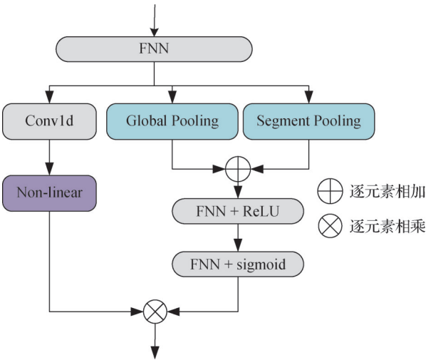
图2 表达增强TDNN网络结构
