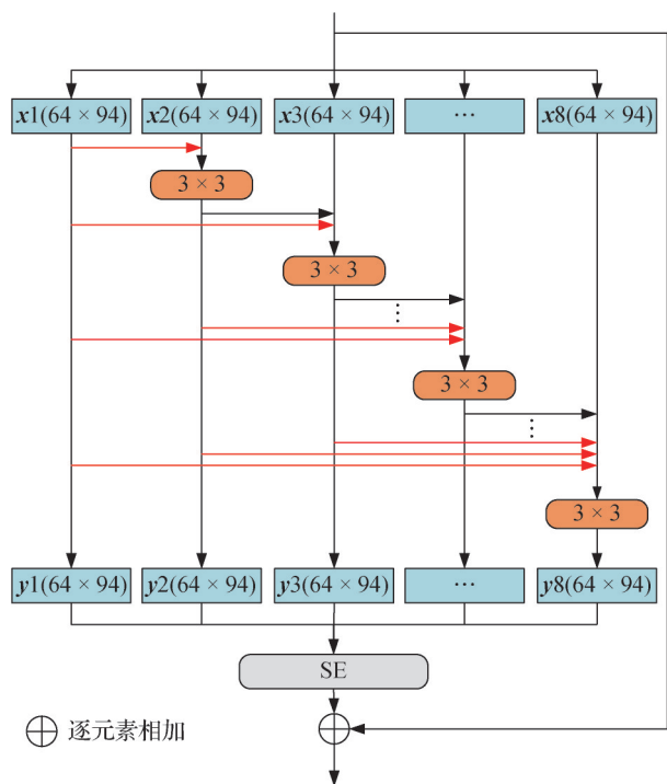
图3 RegB网络结构
