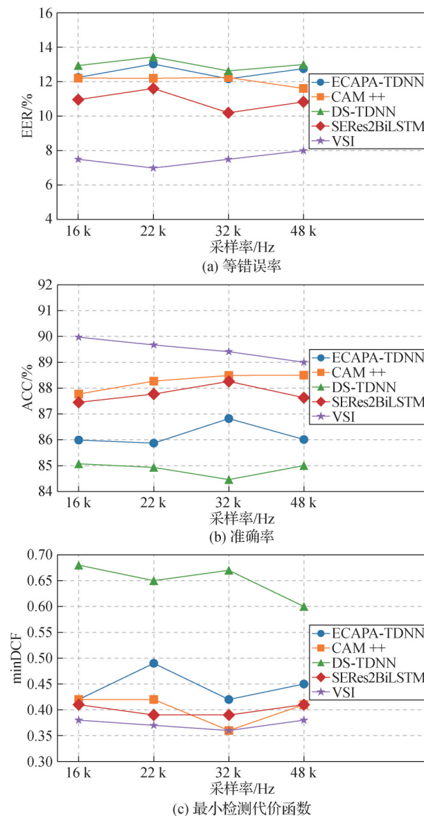
图8 不同采样率下模型指标对比实验结果
