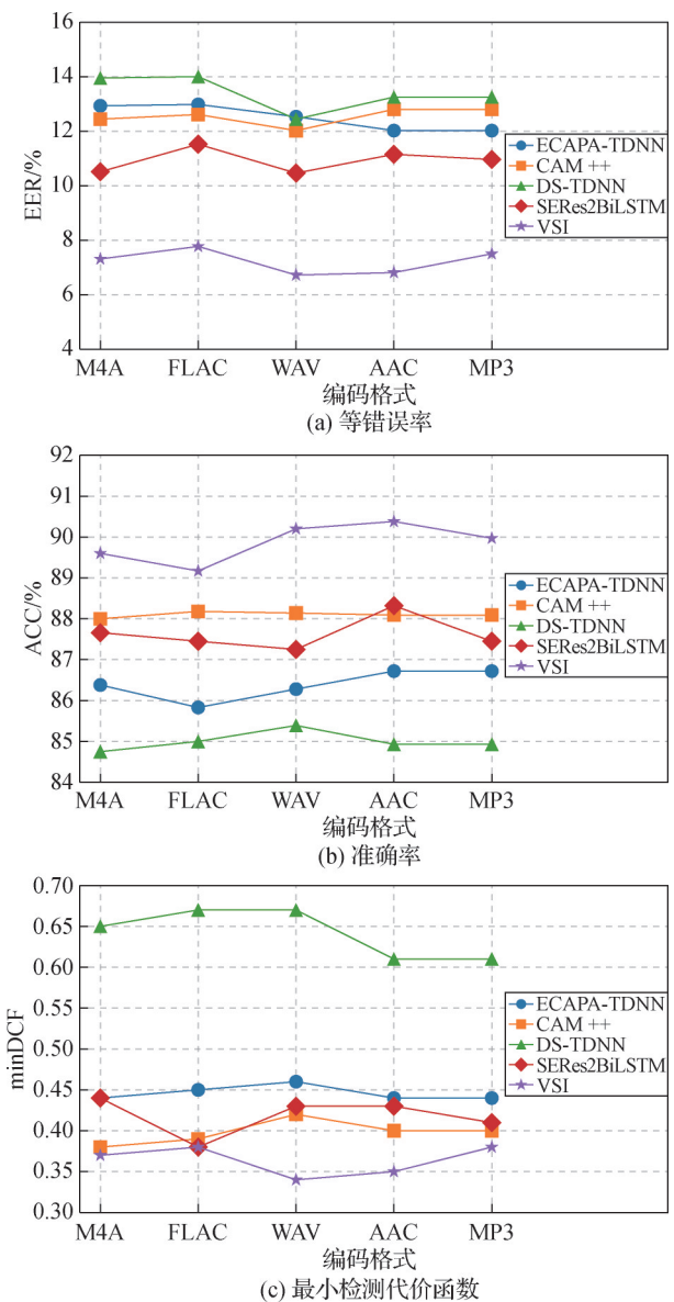
图9 不同编码格式下模型指标对比实验结果
