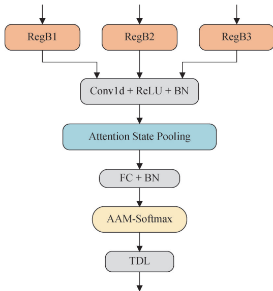
图4 判别网络的模块结构
